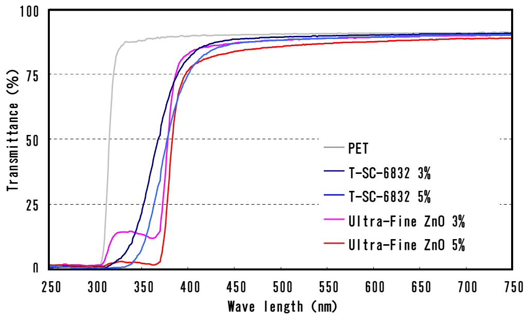
UV遮蔽効果と透明性 [30 \mu m PET Film]
